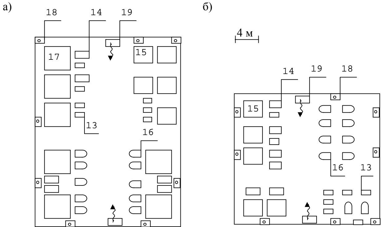
Рис. П.2.4. Расстановка оборудования термического участка
