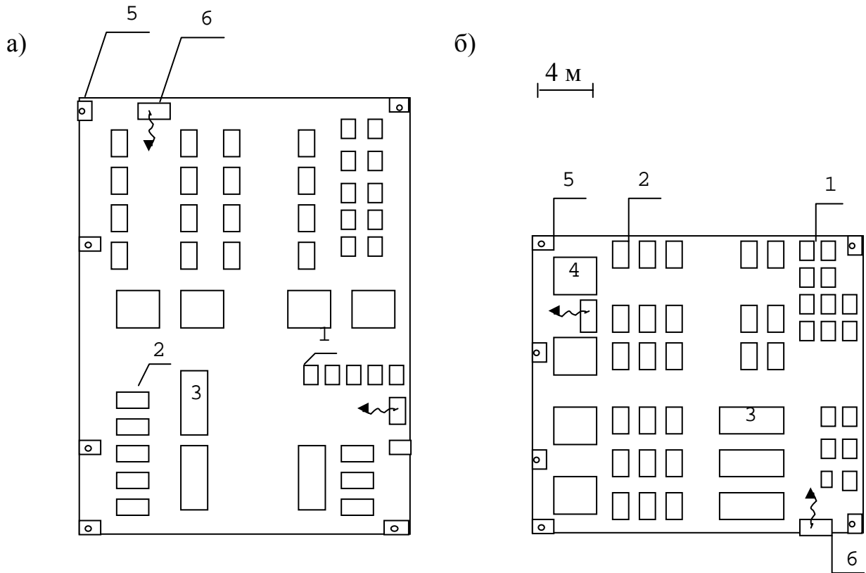
Рис. П.2.2. Расстановка оборудования механического участка
