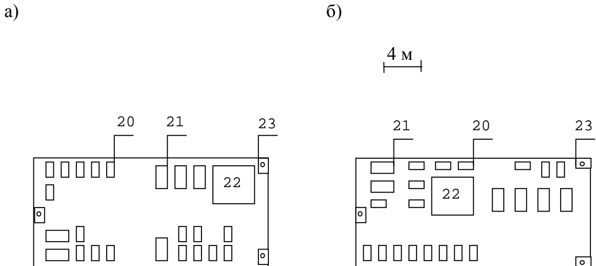
Рис. П.2.5. Расстановка оборудования электроремонтного участка
