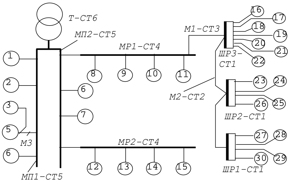
Рис. П.5.1. Расчетная схема цеховой электросети
