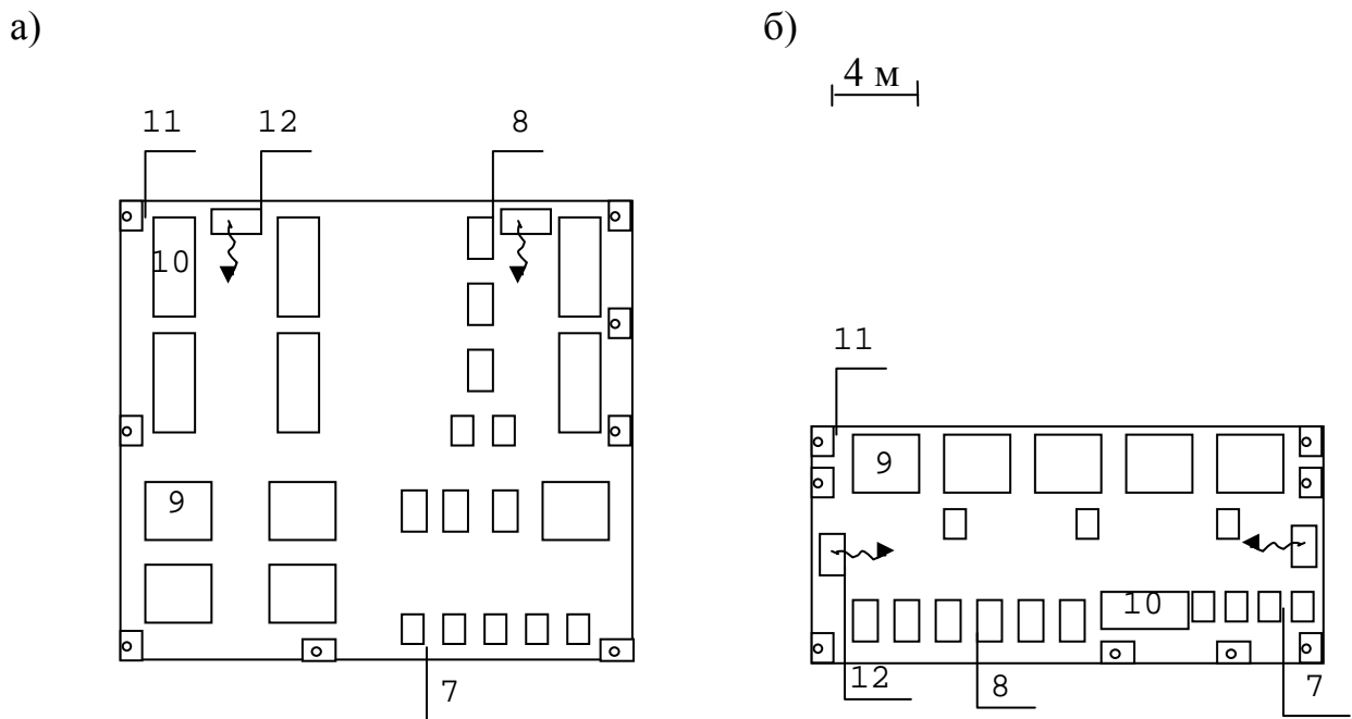
Рис. П.2.3. Расстановка оборудования сварочного участка
